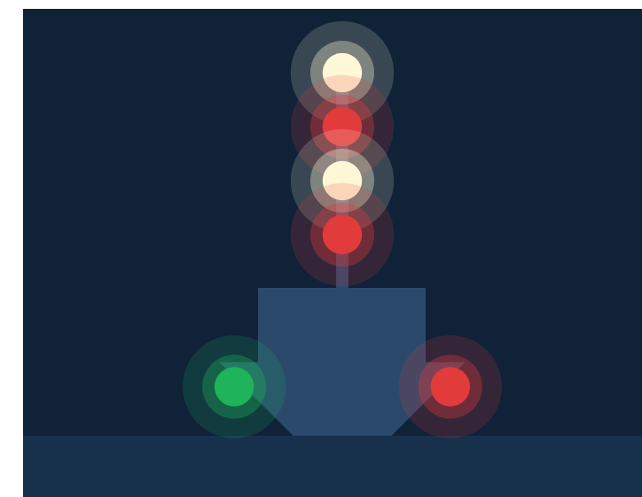
C · Manovrabilità limitata, di prora
